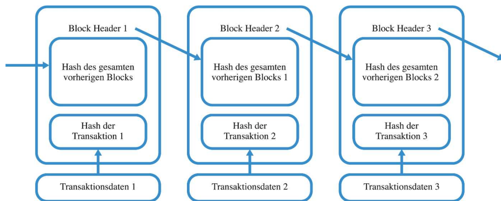
Abbildung 3: Allgemeiner Aufbau einer Blockchain
